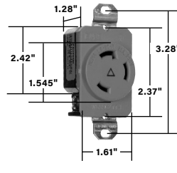
30 Amp Receptacle
