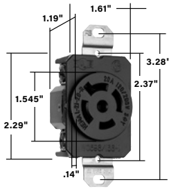
20A Receptacle
